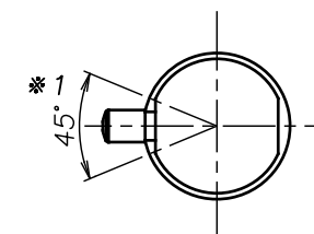
△ A部分矢視図 PARTIAL VIEW A
